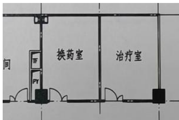
(三)、2 号楼 15 层治疗室及换药室图纸 治疗室：3.9m*5.7m ;换药室：5.4m*5.7m
